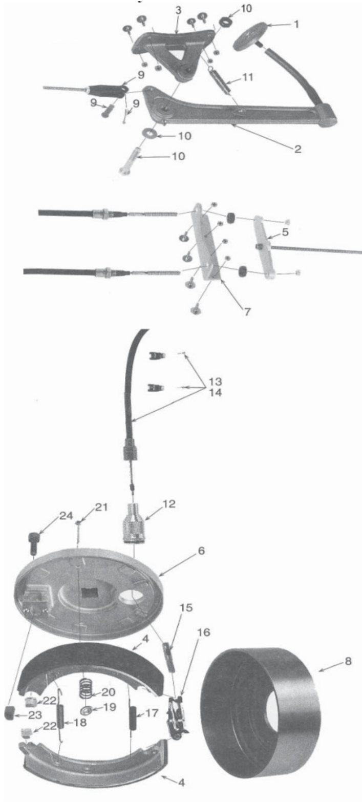
Cable Brake
